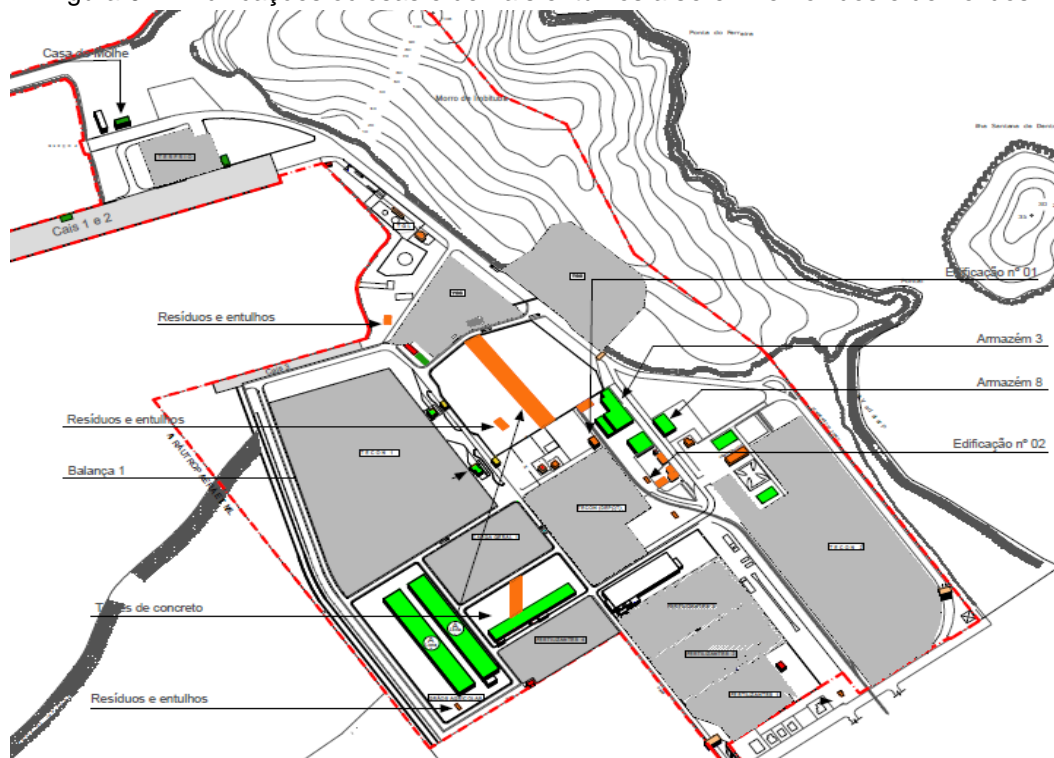
Figura 02 – Edificações ociosas e demais entulhos a serem removidos e demolidos
