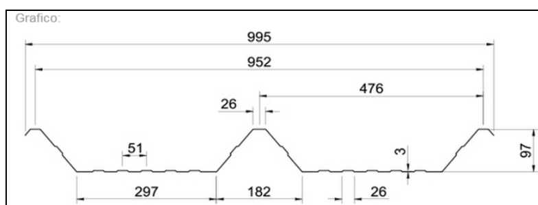
Figura 3 - Dimensões da Telha metálica.
