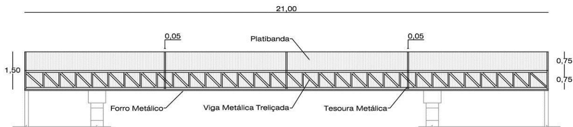
Figura 5 - Corte Transversal da Estrutura
