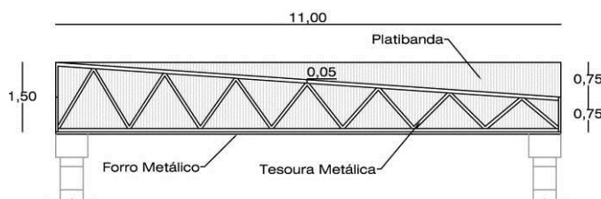
Figura 6 - Corte Longitudinal da Estrutura
