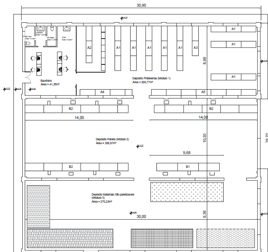
Figura 6 - Layout do Almoxarifado
