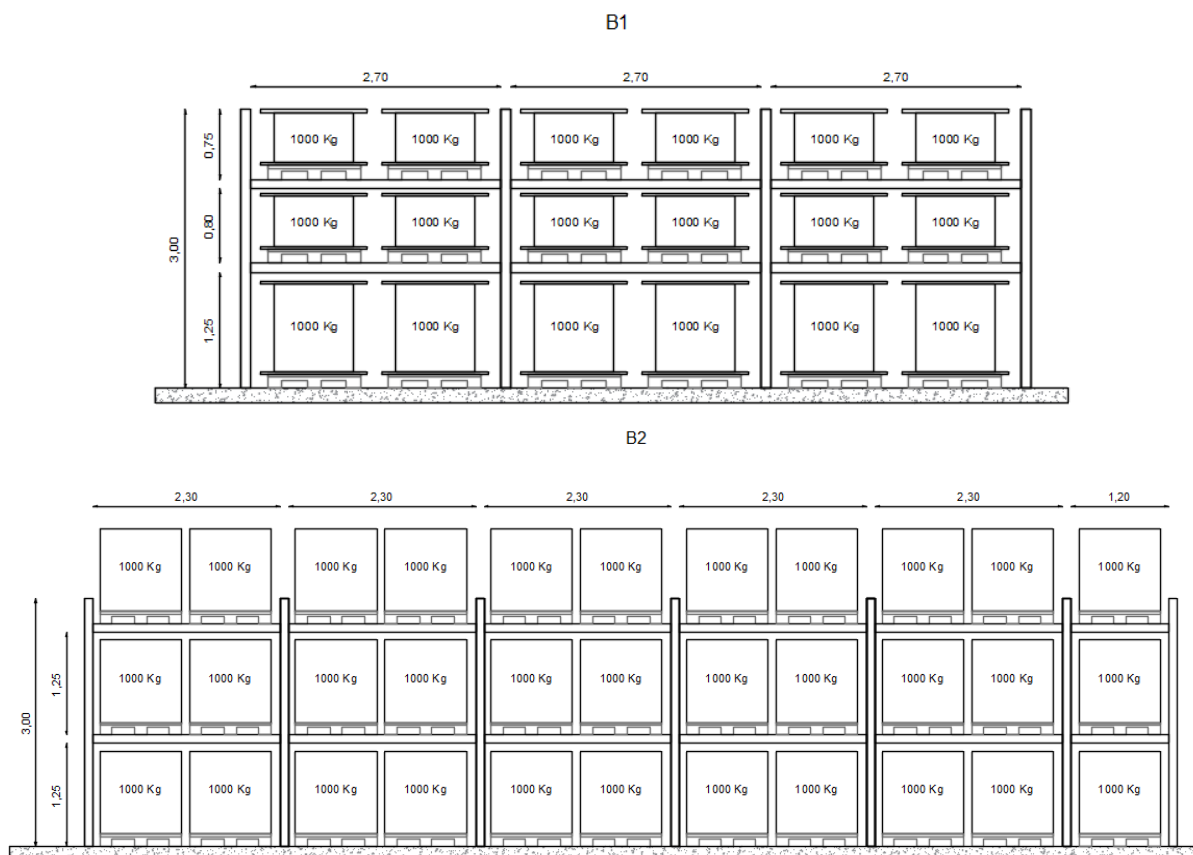
Figura 9 - Orientações para dimensões dos porta paletes
