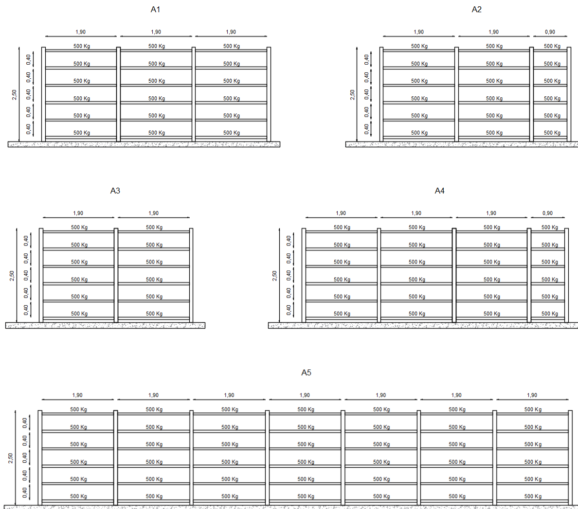
Figura 7 - Orientações para dimensões das Estantes
