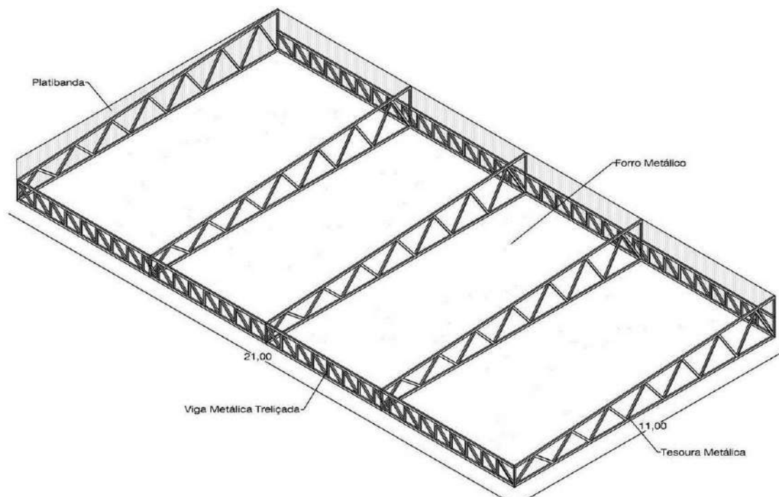
Figura 4 - Detalhe da estrutura metálica a ser recuperada.
