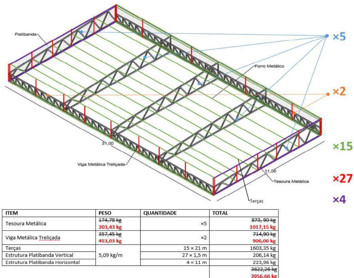
Figura 2 – Identificação da estrutura metálica existente
