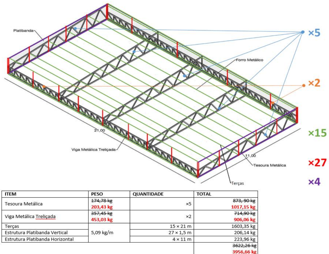
Figura 1: Identificação da estrutura metálica existente
