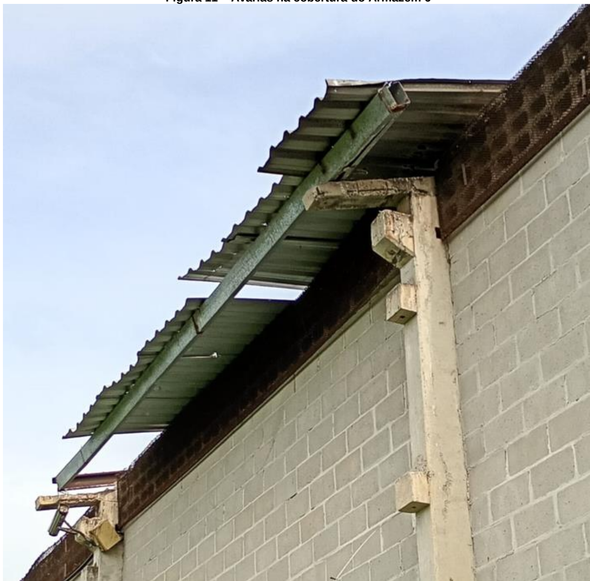
Figura 11 – Avarias na cobertura do Armazém 6
