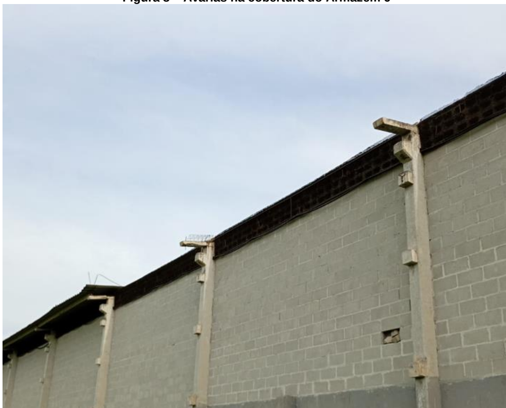
Figura 8 – Avarias na cobertura do Armazém 6
