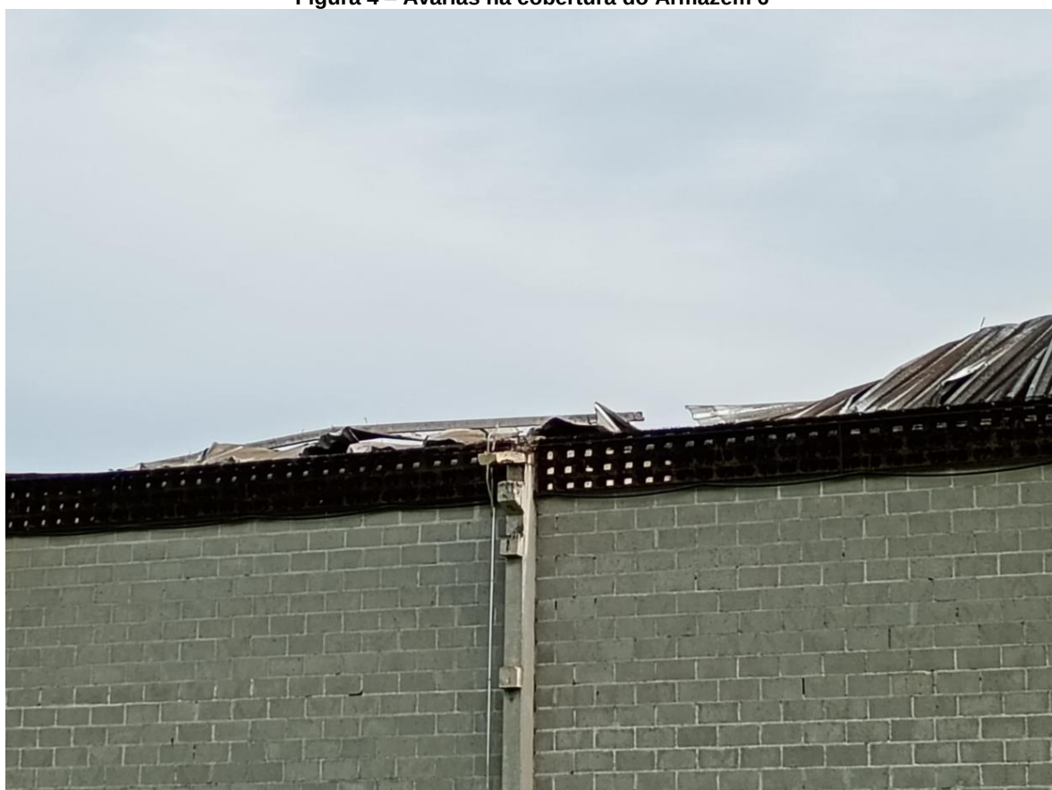
Figura 4 – Avarias na cobertura do Armazém 6
