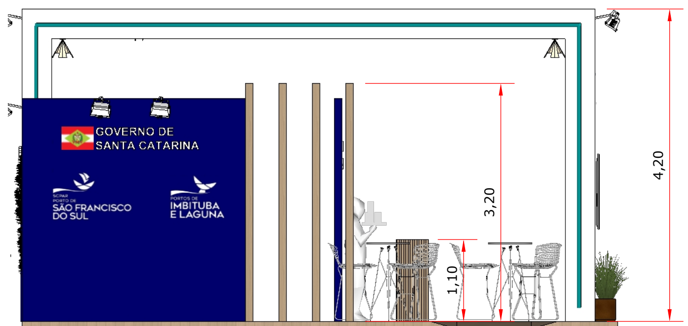
02 VISTA LATERAL ESQ escala 1/50
