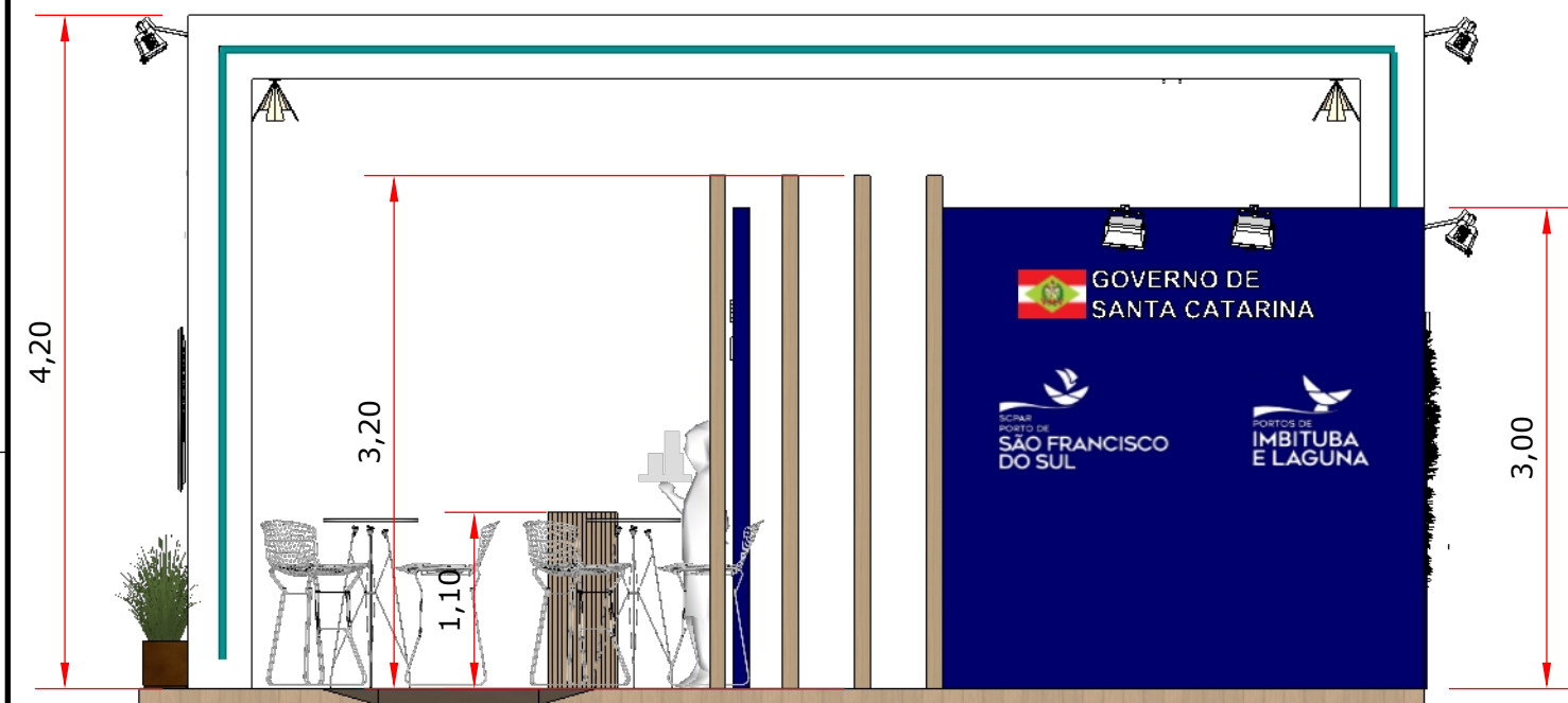
01 VISTA LATERAL DIREITA escala 1/50
