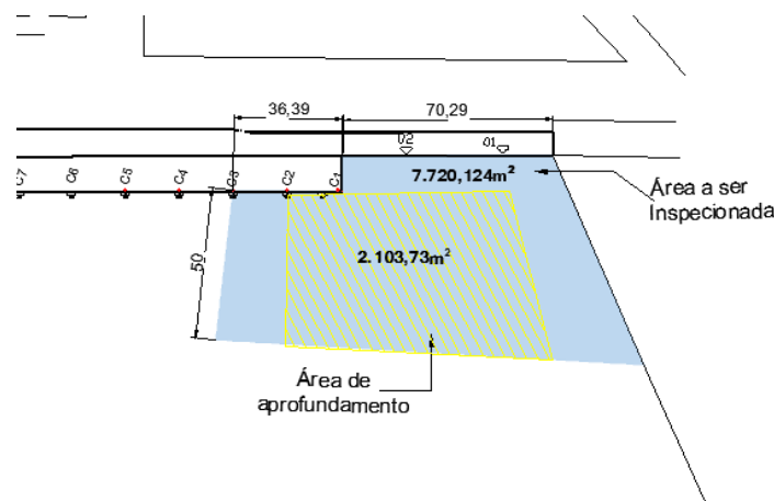
Figura 8 - Área do Cais 1.
