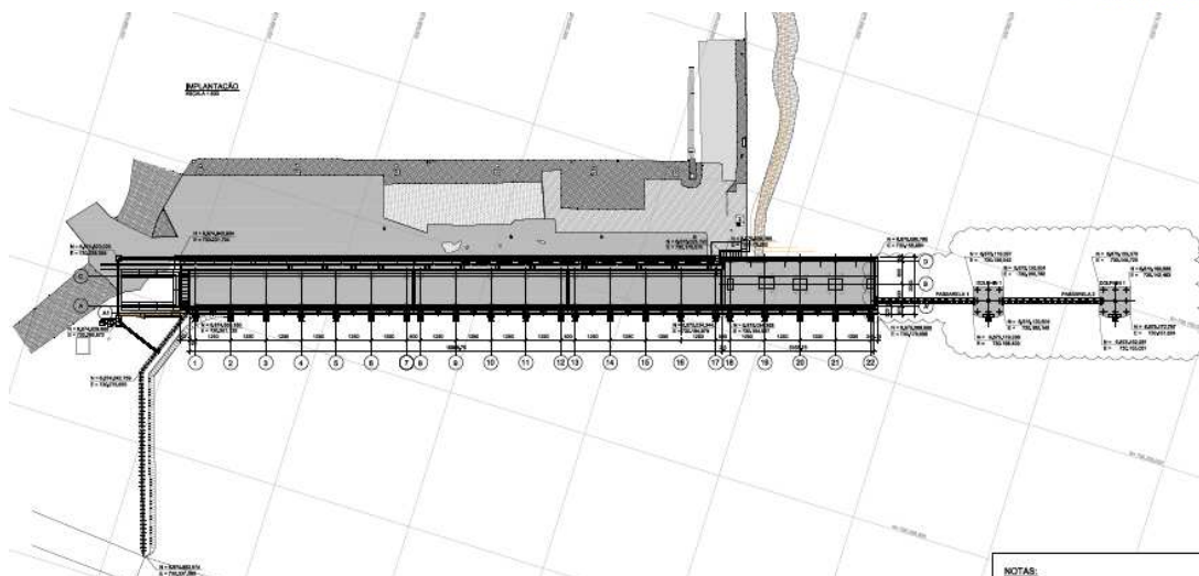
Figura 3 – Planta de implantação referente a obra de Recuperação e Dolphins de Atracação
