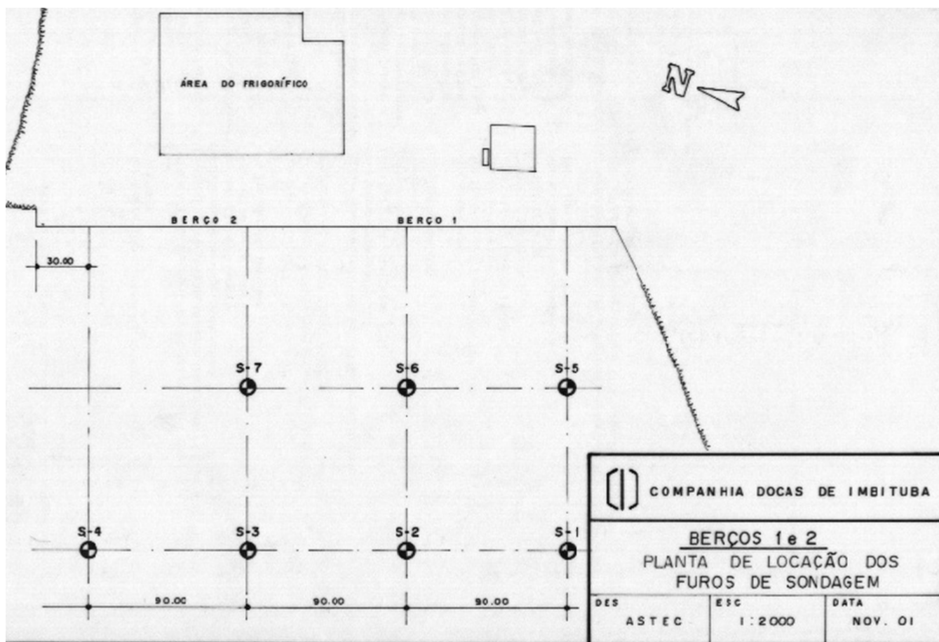
Figura 12 - Planta dos pontos de sondagem
