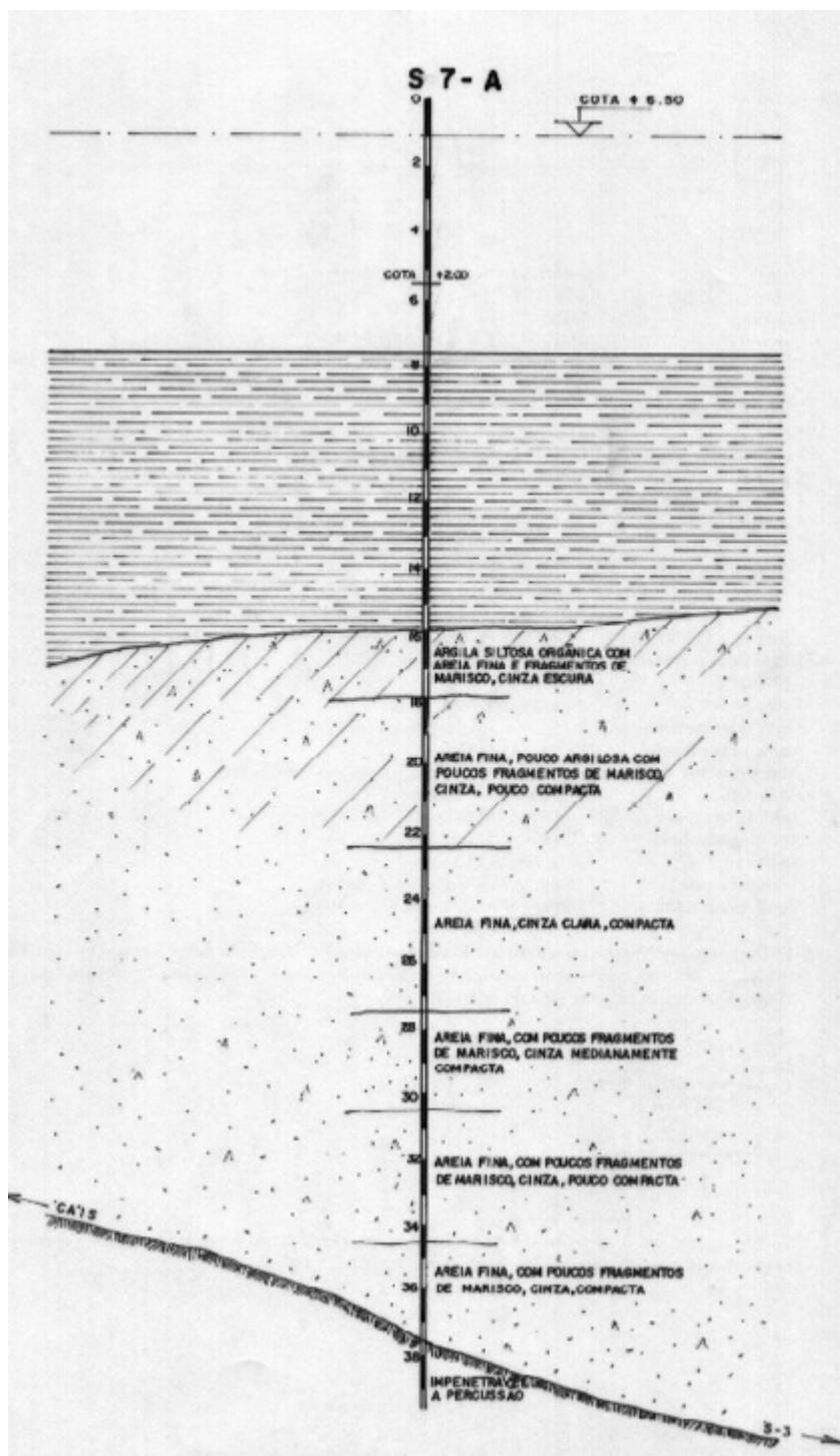
Figura 13 - Caracterização do solo S7-A
