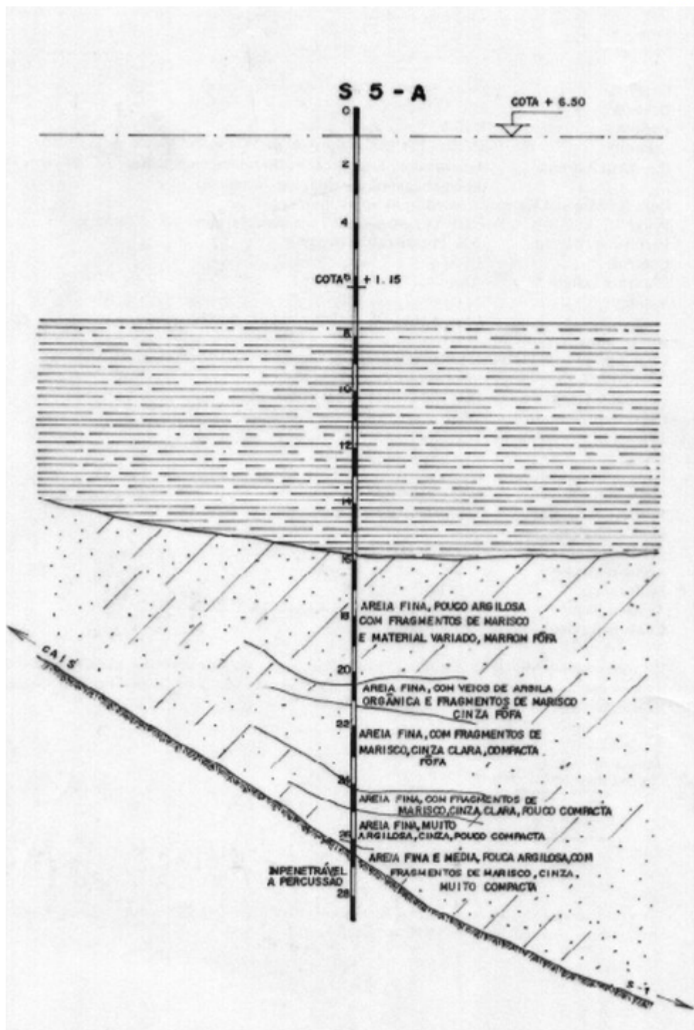
Figura 13 - Caracterização do solo S5-A
