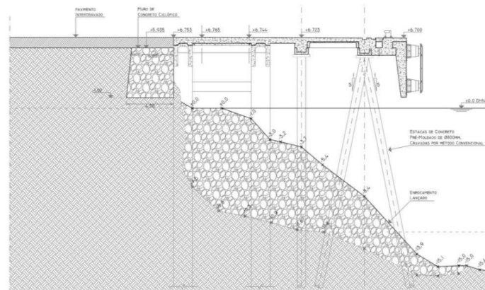
Figura 2 – Cais 1 em corte
