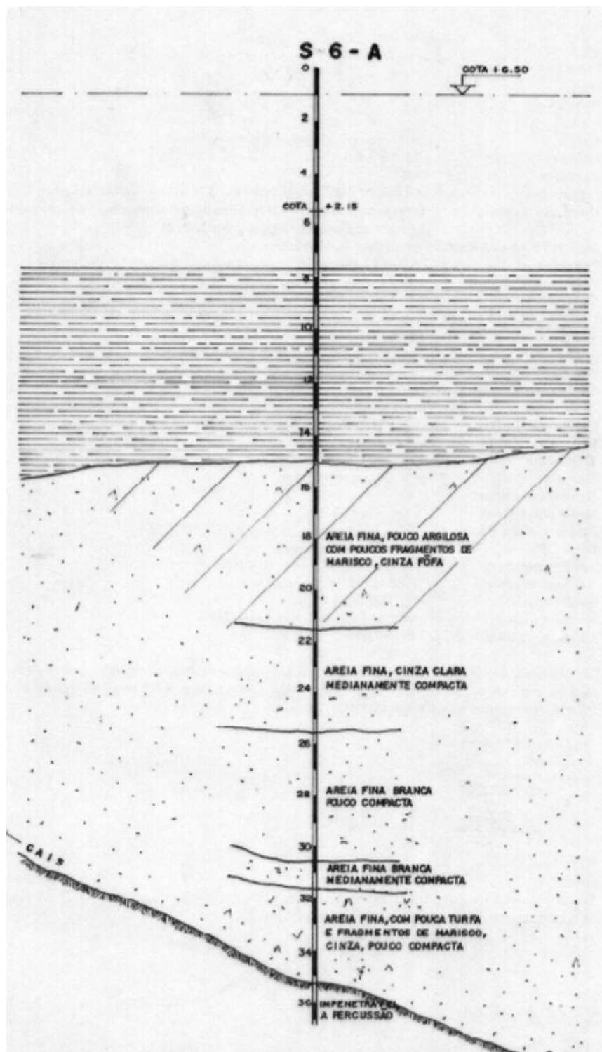
Figura 14 - Caracterização do solo S6-A
