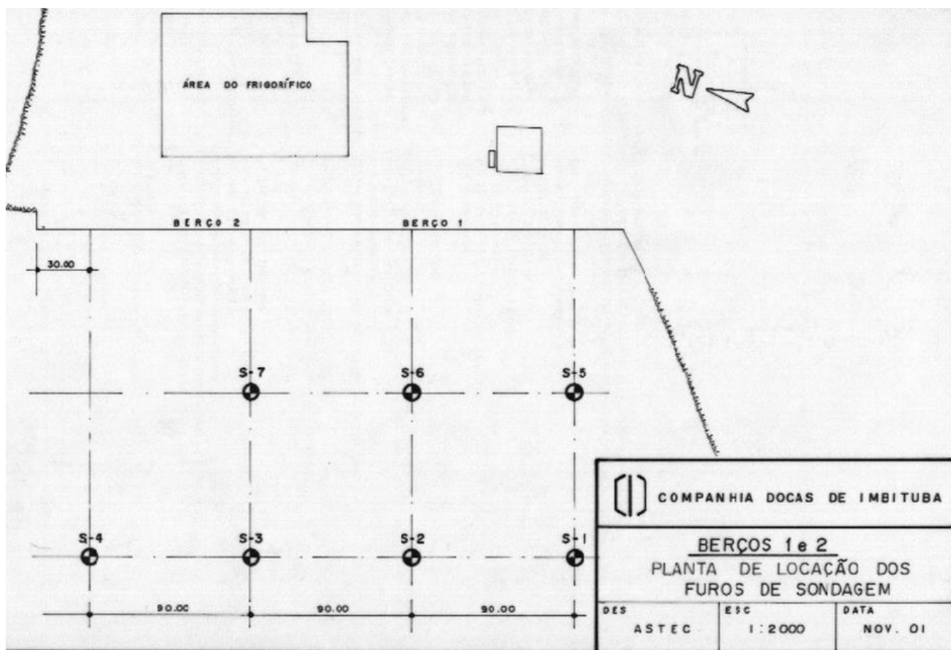
Figura 12 - Planta dos pontos de sondagem
